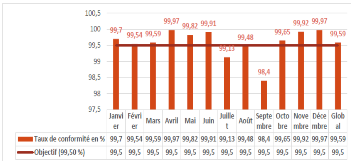
Graphique 2 : Taux global de conformité physicochimique sur l'eau produite par l'ensemble des sites
